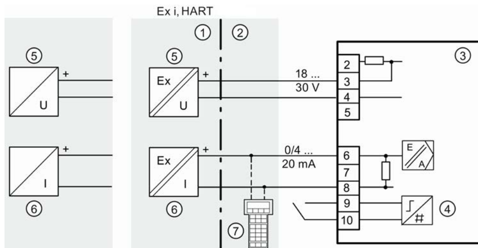
Abb. 29: 4-Leiteranschluss 2/3/4-Leiter-Gerät
