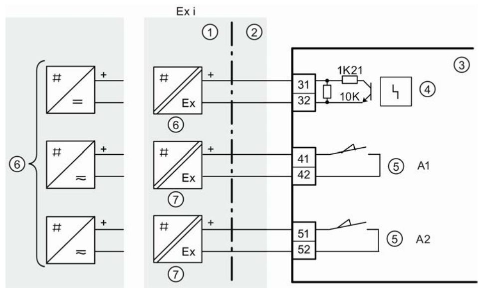
Abb. 36: Kontakt-Modul
