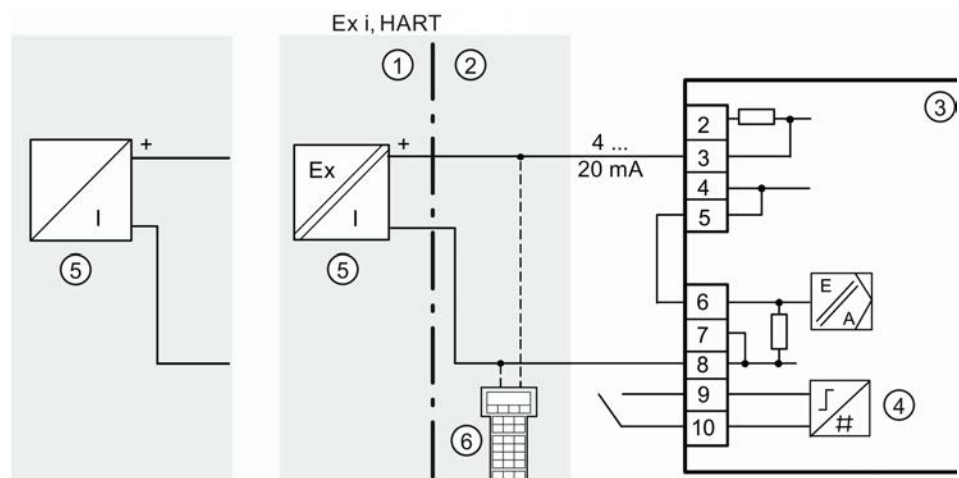
Abb. 27: 2-Leiteranschluss 2/3/4-Leiter-Gerät
