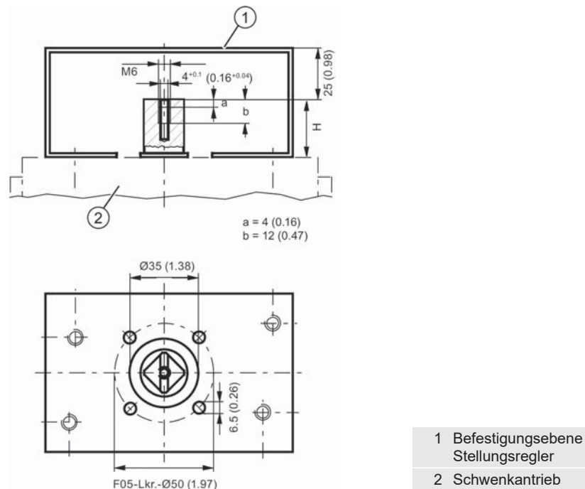
Abb. 23: Anbaukonsole (Lieferung Antriebshersteller) und Maße
