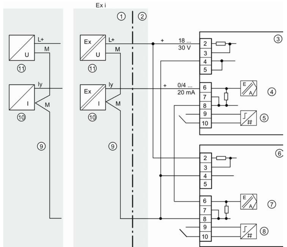
Abb. 30: Reihenschaltung von 2 Stellungsreglern z.B. Split-Range-Betrieb
