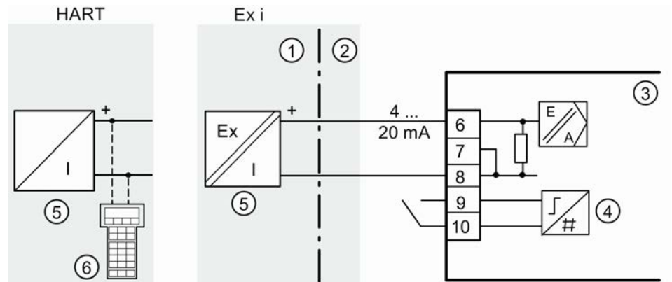
Abb. 26: 2-Leiteranschluss 2-Leiter-Gerät
