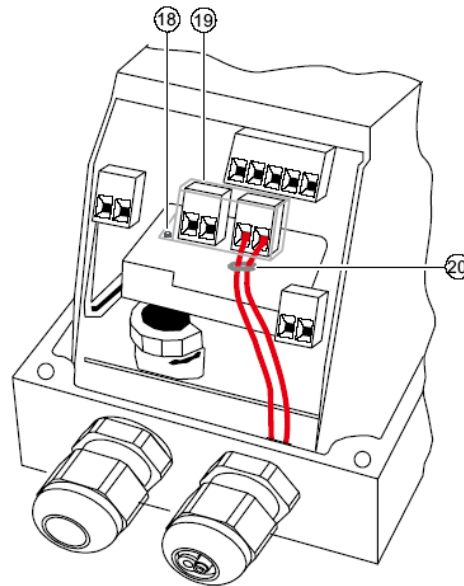
Abb. 35: Kabelbefestigung
