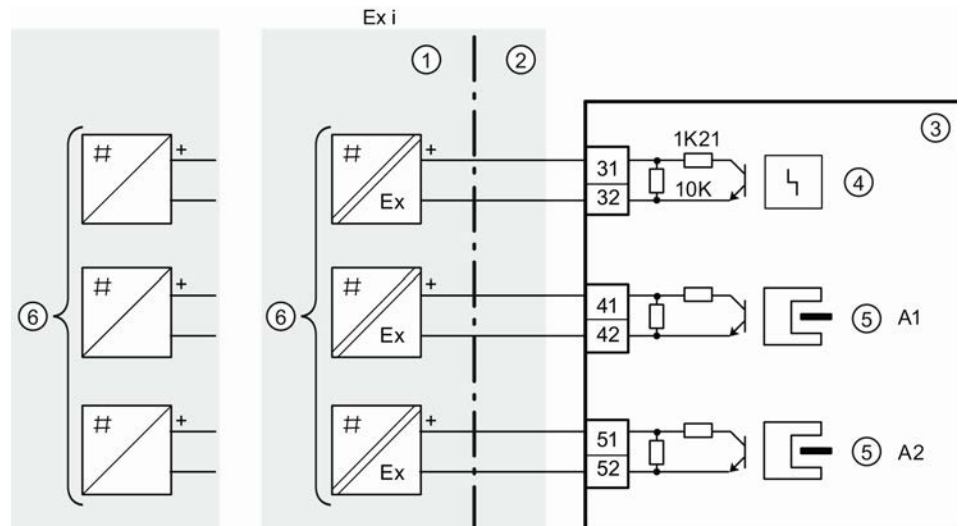
Abb. 34: Schlitzinitiatoren-Modul
