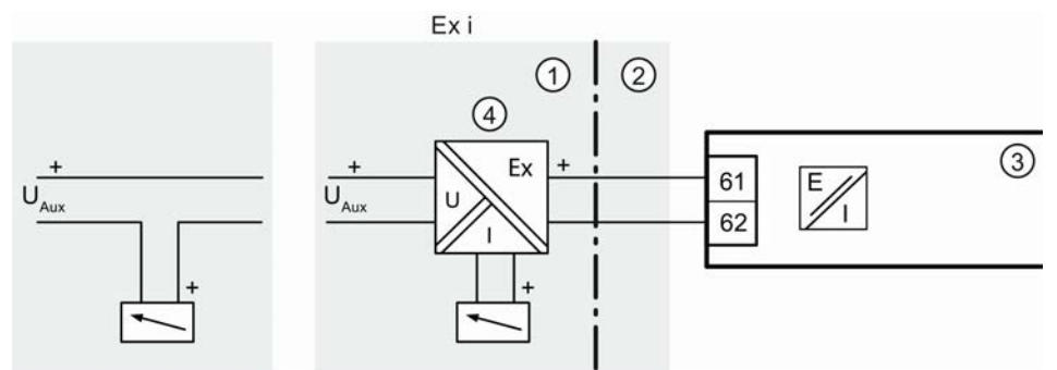
Abb. 31: Analog-Modul
