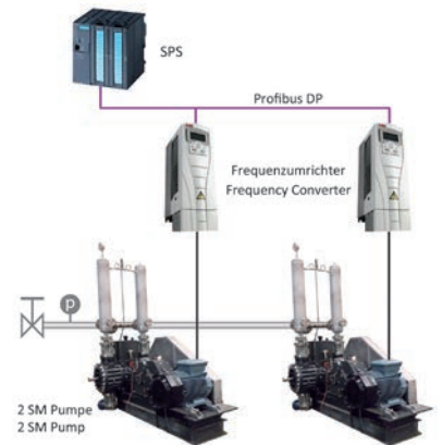
Abb. 2: Kurbelwellenkopplung zweier doppelt wirkenden Einzylinderpumpen..
