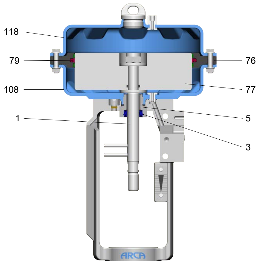
Abb. 6: Schnittbild
